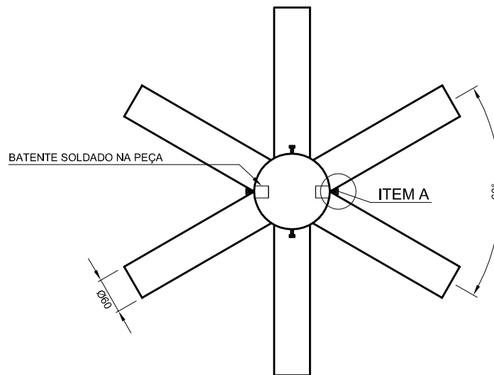
VISTA SUPERIOR
