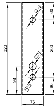
VISTA FRONTAL DA BASE DO BRAÇO CURTO Esp.: 3,00mm
