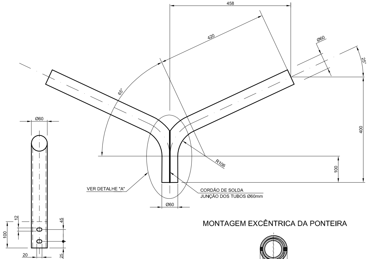
DETALHE "A"
