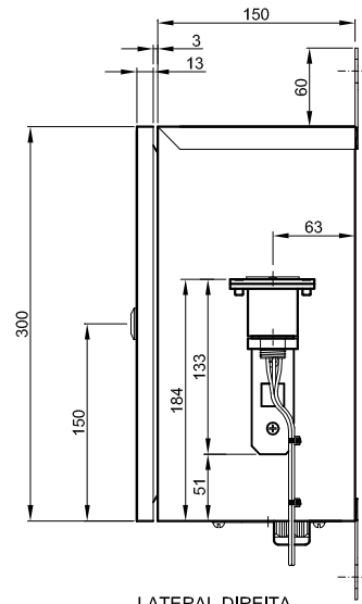
LATERAL DIREITA
