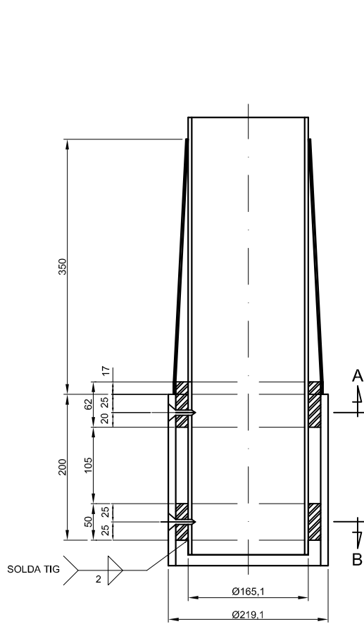
DETALHE DA JUNÇÃO
