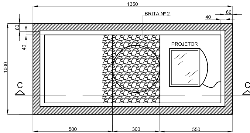
VISTA SUPERIOR SEM GRADE
