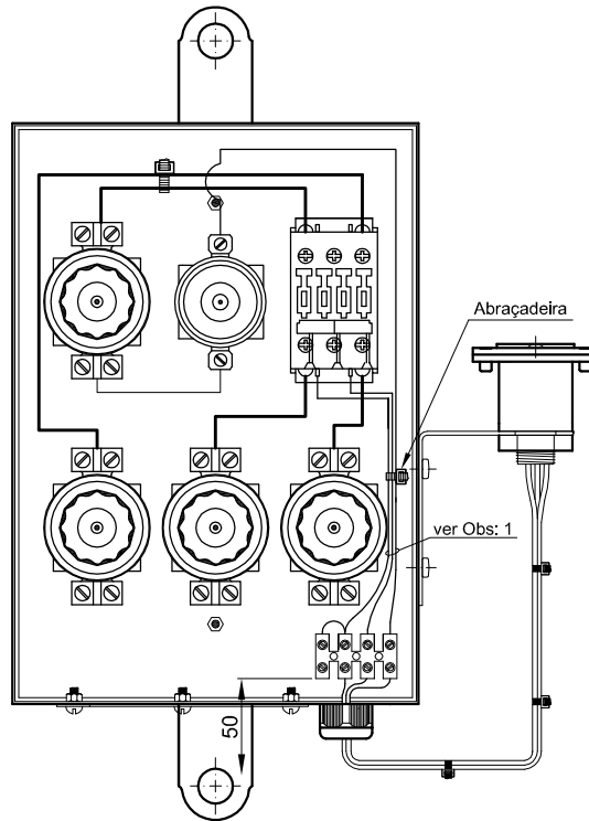
VISTA INTERNA
