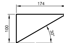
VISTA FRONTAL DO TRIANGULO DO BRAÇO CURTO Esp.: 3,00mm
