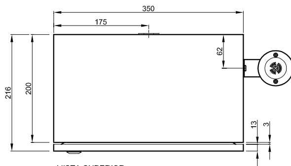
VISTA SUPERIOR
