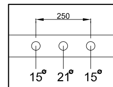
DETALHE DA FURAÇÃO PARA FIXAÇÃO DO PROJETOR NA BASE DE ALVENARIA
