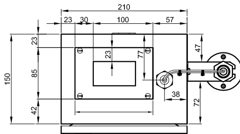
VISTA INFERIOR
