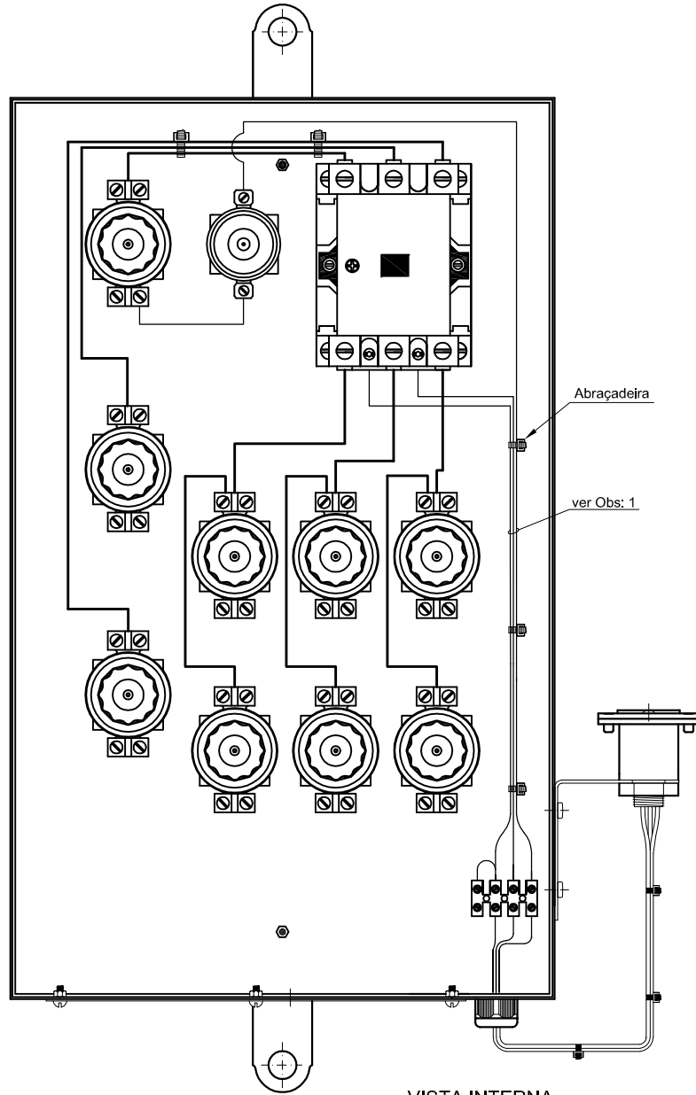
VISTA INTERNA
